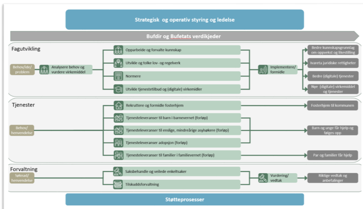
Figur: Virksomhetsmodell
