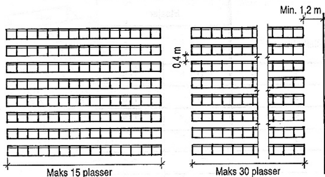
§ 7-27 fig 21 Forsamlingslokaler innredet med sitteplasser
