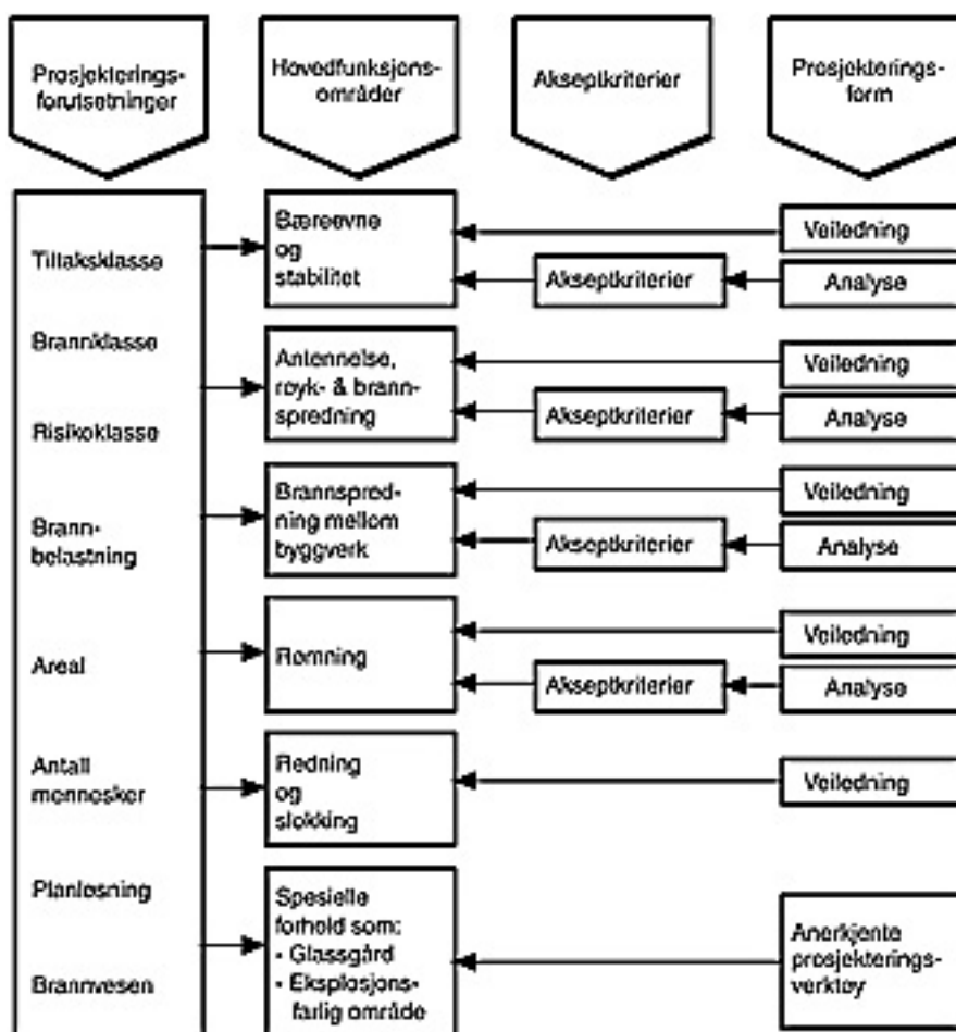
§ 7-21 fig 1 Hovedelementer i den branntekniske prosjektering
