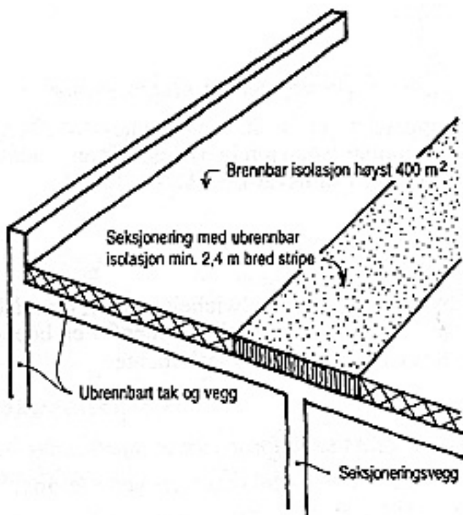
§ 7-24 fig 6 Tekkedetaljer ved tilslutninger og gjennomføringer
