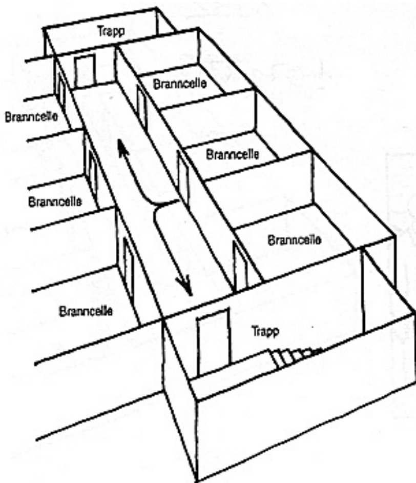
§ 7-27 fig 20 Branncelle med utgang til to trapperom utført som rømningsvei
