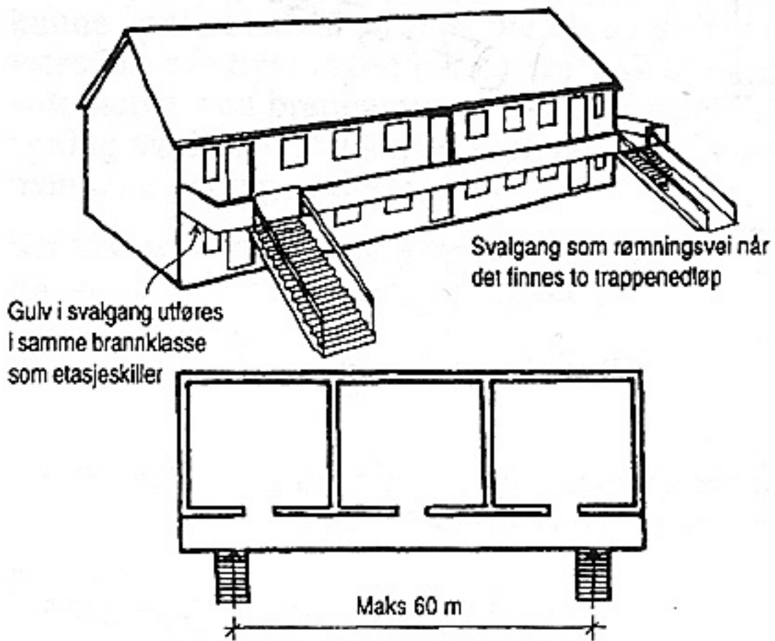
§ 7-27 fig 24 Brannbeskyttelse av rømningstrapp fra svalgang
