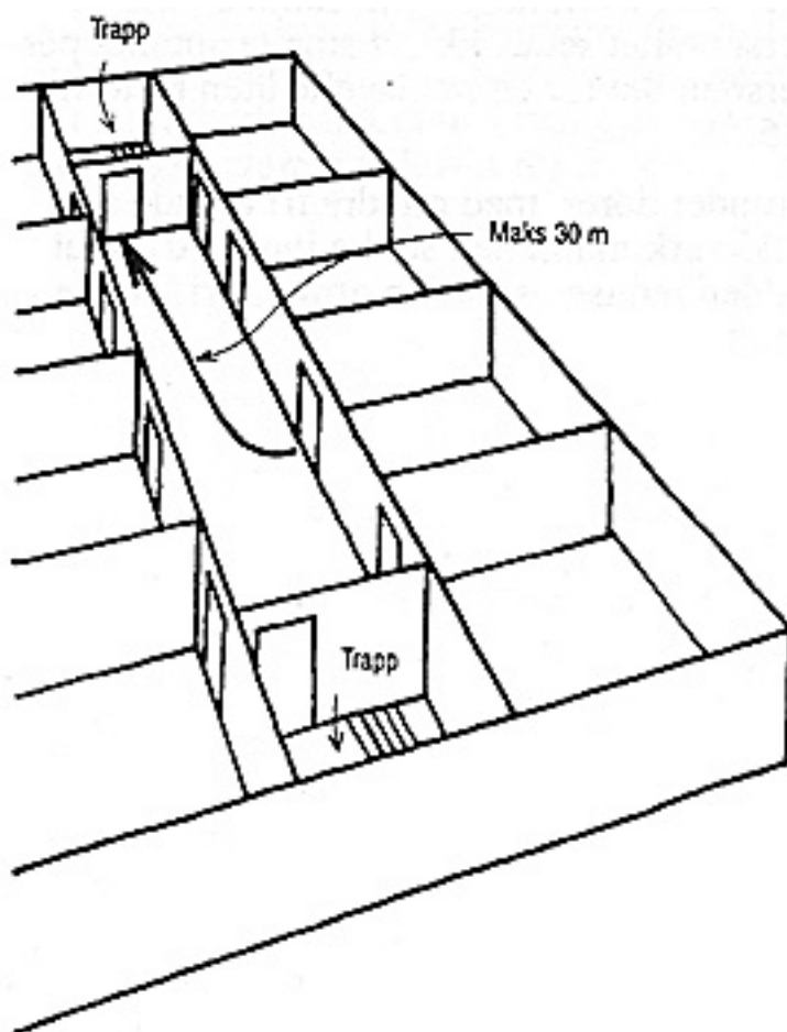
§ 7-27 fig 17 Avstand fra dør i branncelle til nærmeste trapp/utgang når det finnes bare en trapp eller utgang eller når vindu utgjør den ene av to rømningsveier
